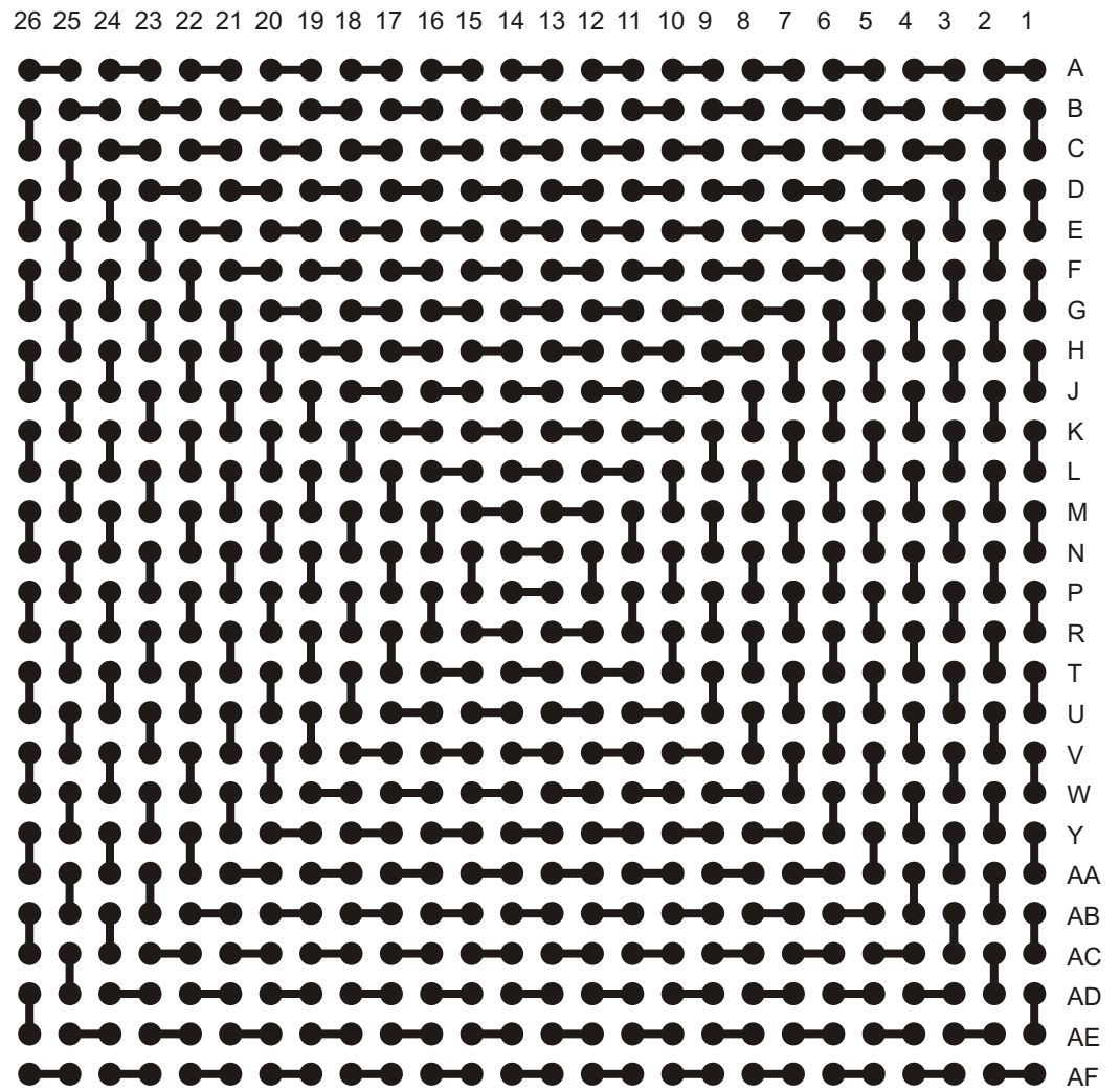
PBGA676-1.0mm-27mm-DC
