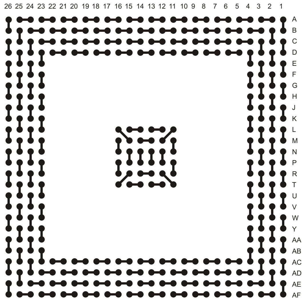
A-PBGA388-1.27mm-35mm-DC
