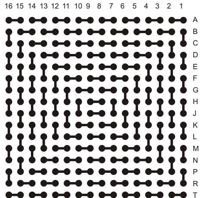
A-PBGA256-1.0mm-17mm
