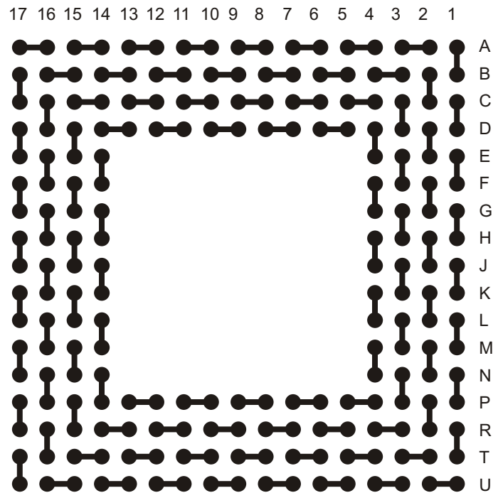
A-CABGA208-.8mm-15mm-DC
