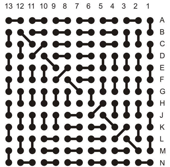
PBGA169-1.5mm-23mm-DC
