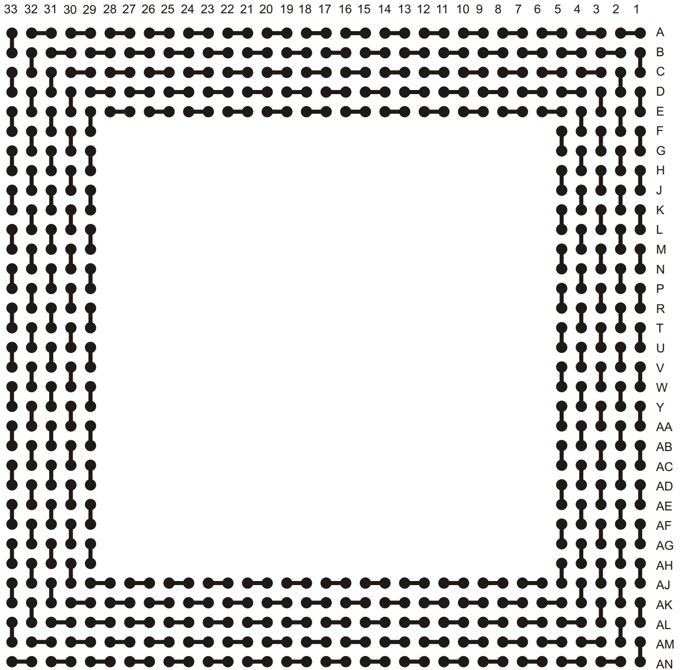
A-SBGA560-1.27mm-42.5mm-DC
