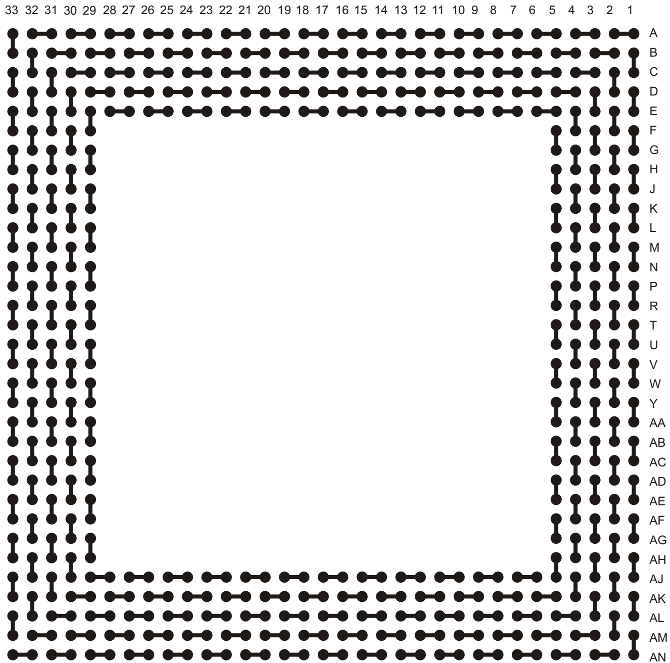
A-SBGA560-1.27mm-42.5mm-DC
