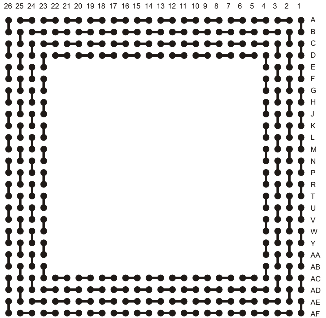
A-SBGA352-1.27mm-35mm-DC
