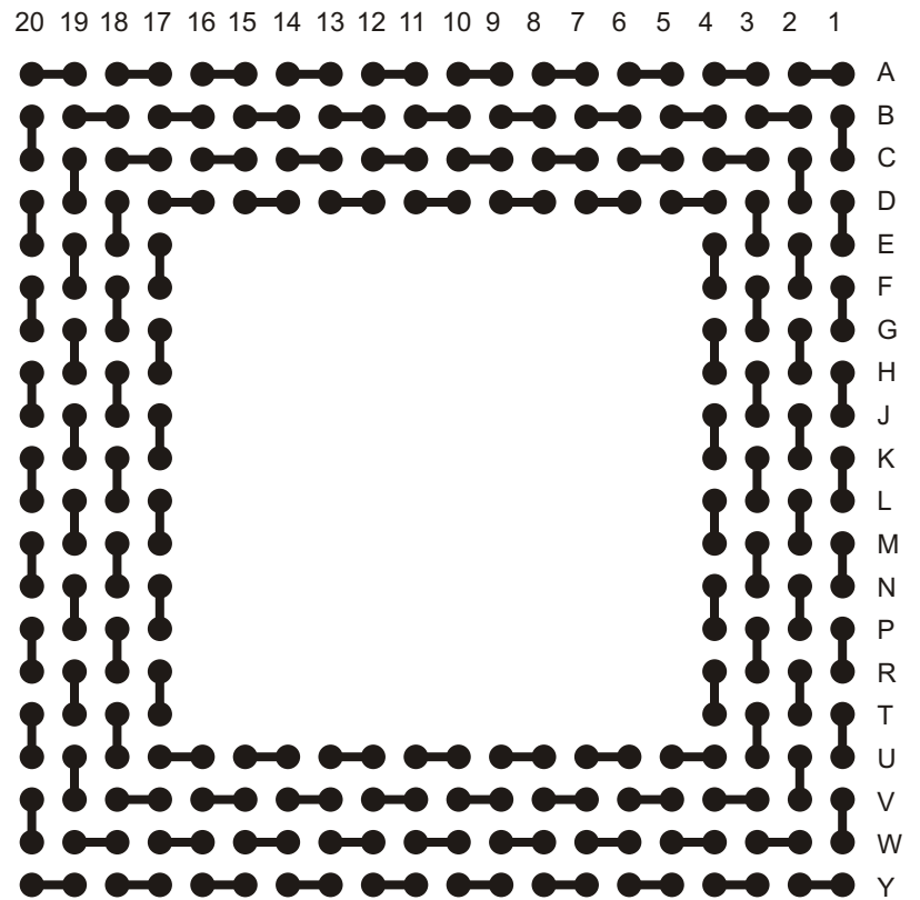
A-SBGA256-1.27mm-27mm-DC
