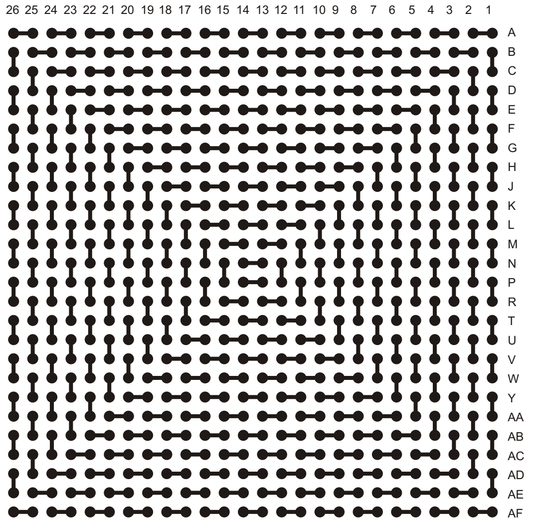
PBGA676-1.0mm-27mm-DC
