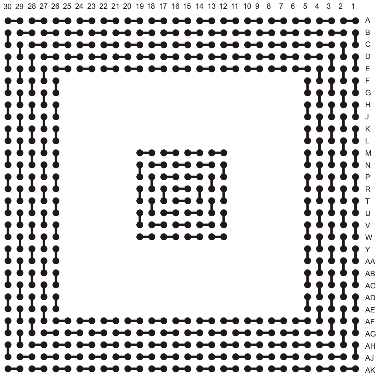
A-PBGA564-1.27mm-40mm-DC
