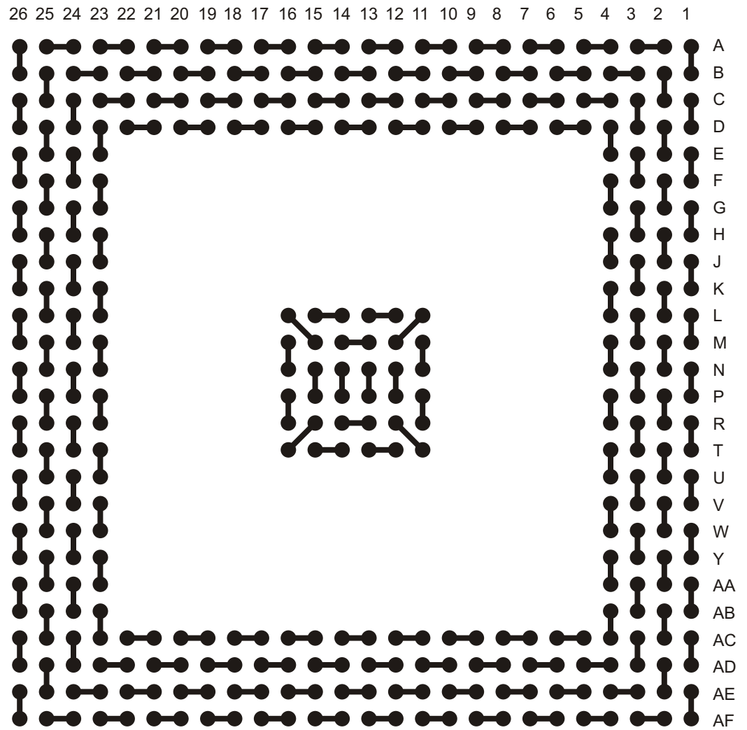
A-PBGA388-1.27mm-35mm-DC
