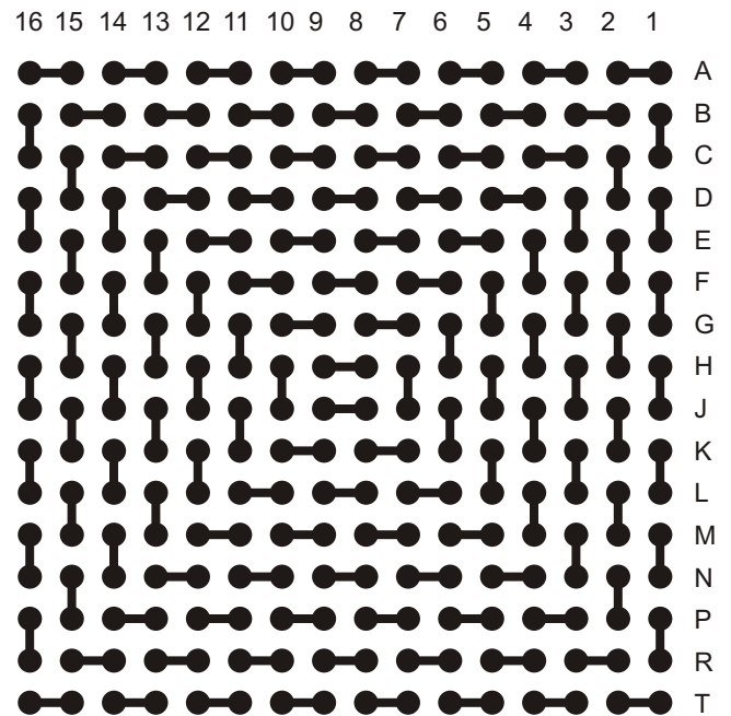
A-PBGA256-1.0mm-17mm
